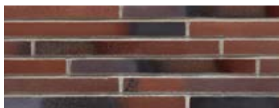
455 braun-blau 490 x 40 x 14 mm \Delta < 3\% DIN EN 14411, Gr. AI b
