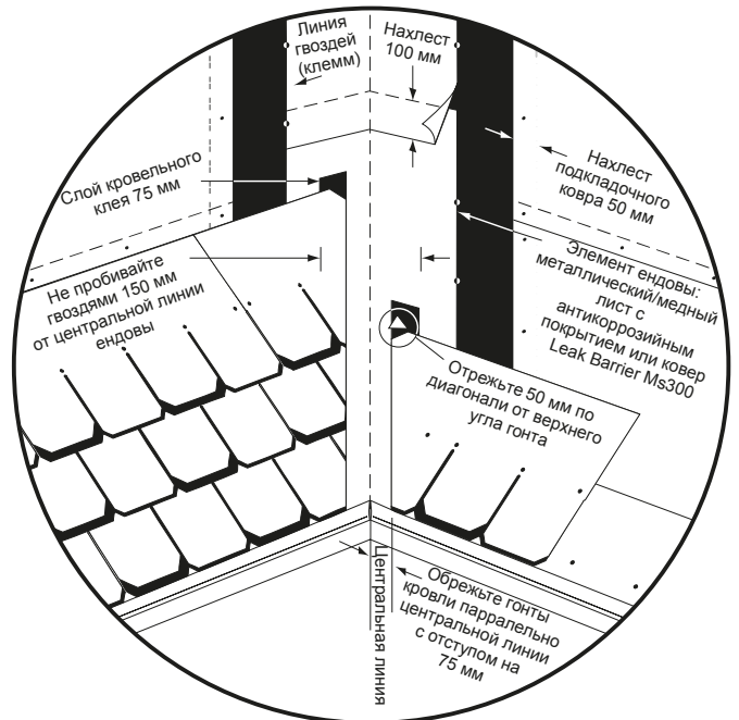
Рисунок 17-11. Устройство ендовы для Grand Manor и Belmont
